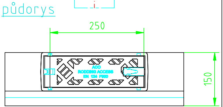
KerbDrain 305 těleso žlabu, délka 0,5m, s revizním otvorem , obj. číslo 07962
