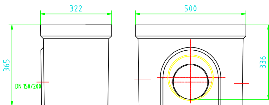
spodní díl krátký tvar obj. číslo 01614/ DN150 obj. číslo 06190/ DN200
