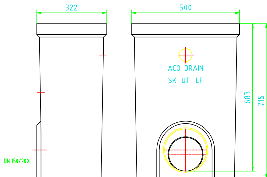
spodní díl hluboký tvar obj. číslo 03217/ DN150 obj. číslo 08565/ DN200
