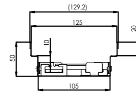
Ansicht Baubreite 130mm
