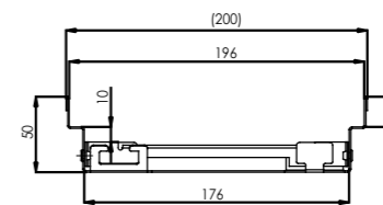
Ansicht Baubreite 200mm
