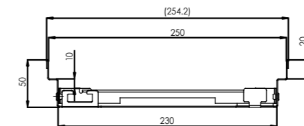
Ansicht Baubreite 250mm
