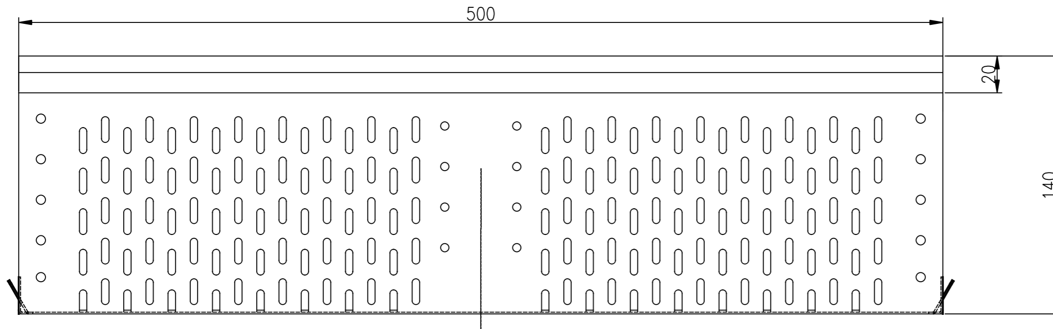
Ansicht Variante 1
