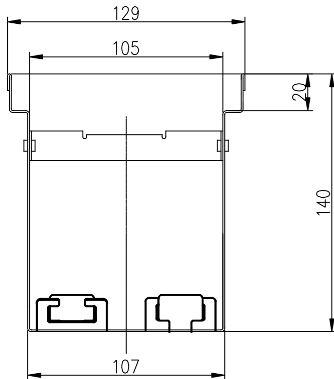
Schnitt Variante 1
