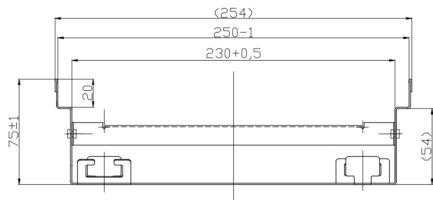
Ansicht Baubreite 250mm (M 2:1)
