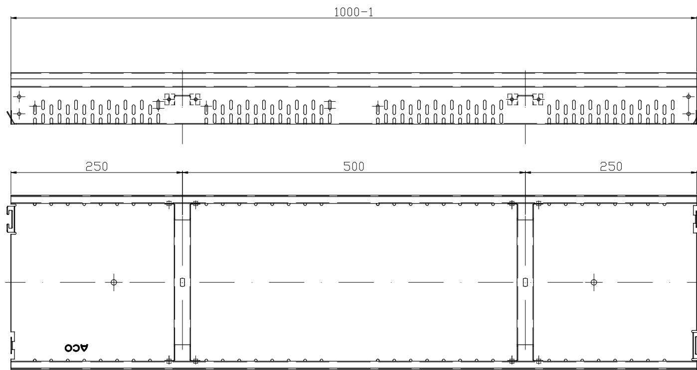
Ansicht Baubreite 250mm (M 2:1)
